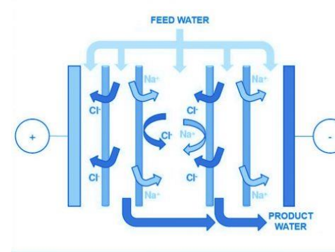
Electrodeionization
